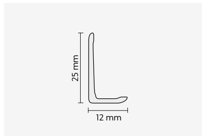
WIDOCZNY, 1 - CZĘŚCIOWY Profil końcowy „L” - duży
