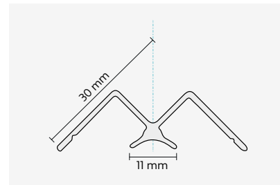
WIDOCZNY, 1 - CZĘŚCIOWY Profil narożny wewnętrzny 90°
