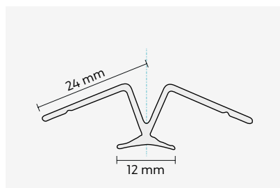
WIDOCZNY, 1 - CZĘŚCIOWY Profil narożny wewnętrzny 135°
