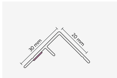
UKRYTY, 1 - CZĘŚCIOWY Profil narożny wewnętrzny 90°
