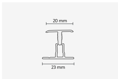
WIDOCZNY, 2 - CZĘŚCIOWY Profil łączący
