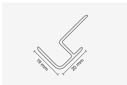
WIDOCZNY, 1 - CZĘŚCIOWY Profil narożny zewnętrzny 90°
