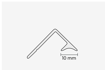
COMBI Profil narożny wewnętrzny 90°
