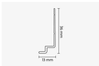
ALU Profil startowy
