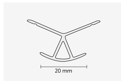
WIDOCZNY, 1 - CZĘŚCIOWY Profil narożny zewnętrzny 135°
